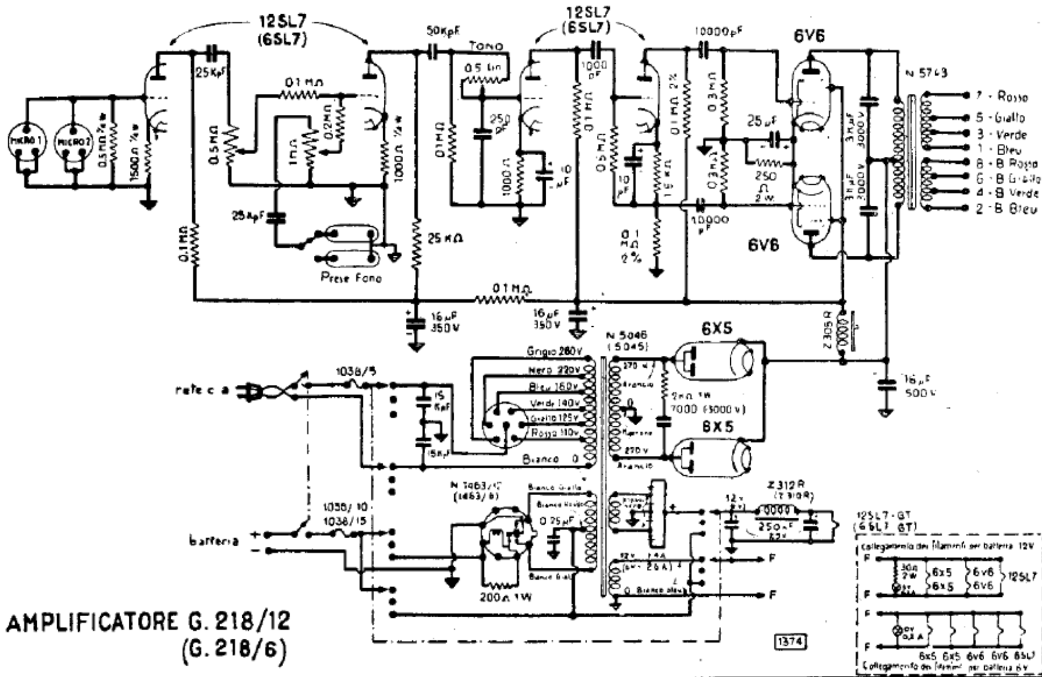
Lo schema elettrico del G. 218. - Le indicazioni dei collegamenti dei filamenti nei due tipi sono indicate nei piccoli schemi in basso a destra.
